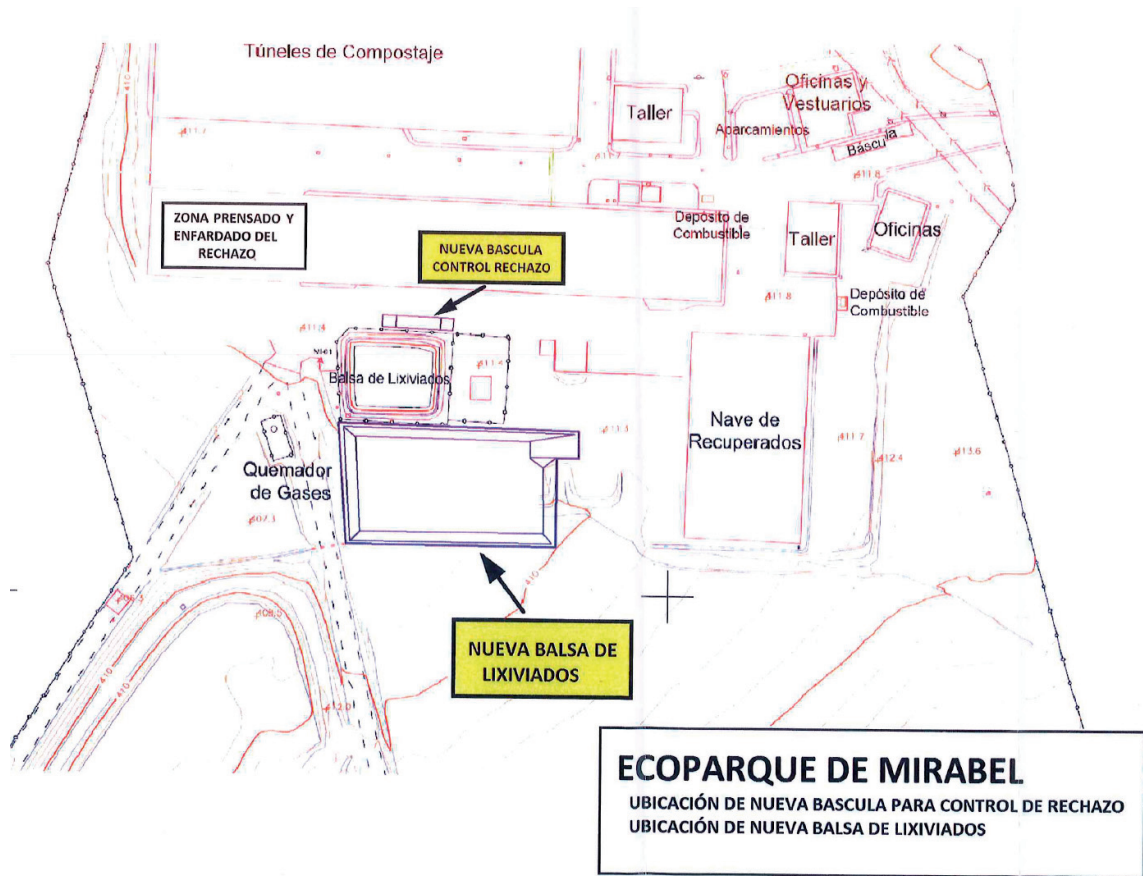
Figura 1. Plano 1 en planta de la instalación. Zona de tratamiento.
