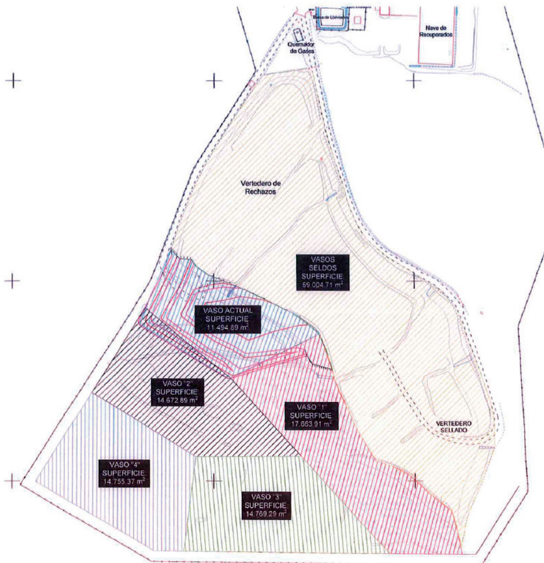
Figura 2. Plano 2 en planta de la instalación. Zona de vasos de vertido.
